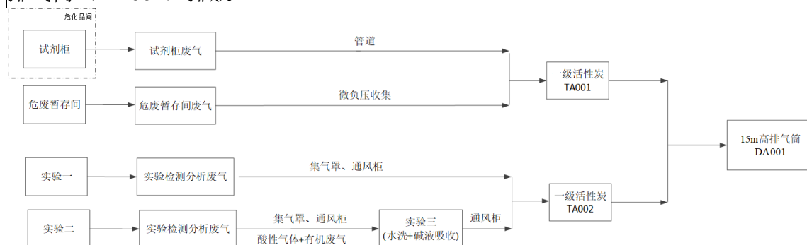
图 4-1 废气治理流程图
