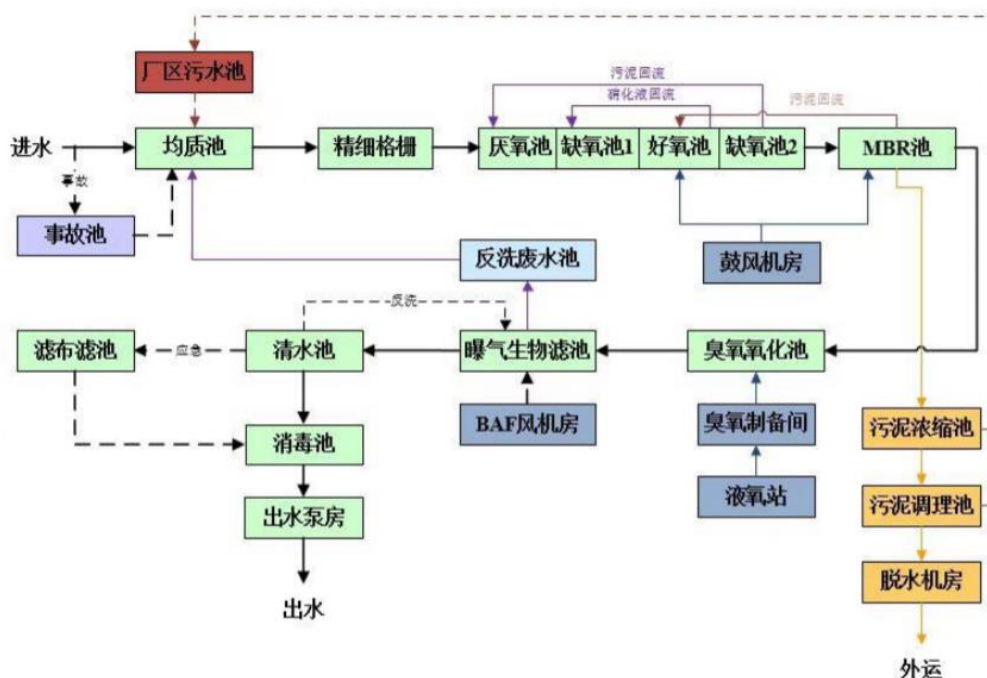
图 4-2 改造后污水处理厂二期工程污水处理流程图
